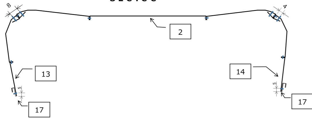
SEC : C-C
