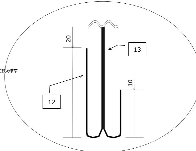
DETAIL : D
