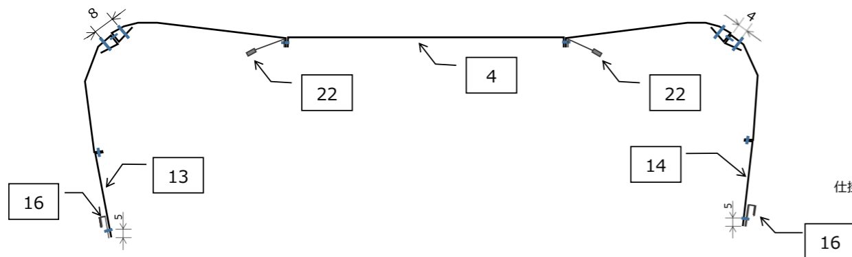
SEC : B-B
